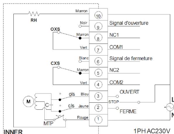
SCHEMA DE CÂBLAGE
